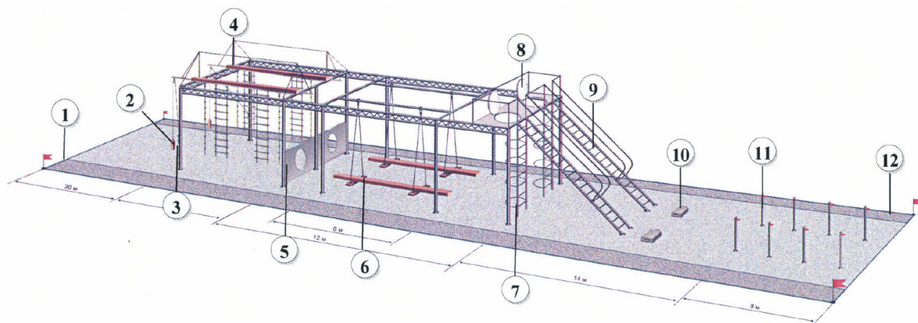
Рис. 47. Схема морской полосы препятствий
