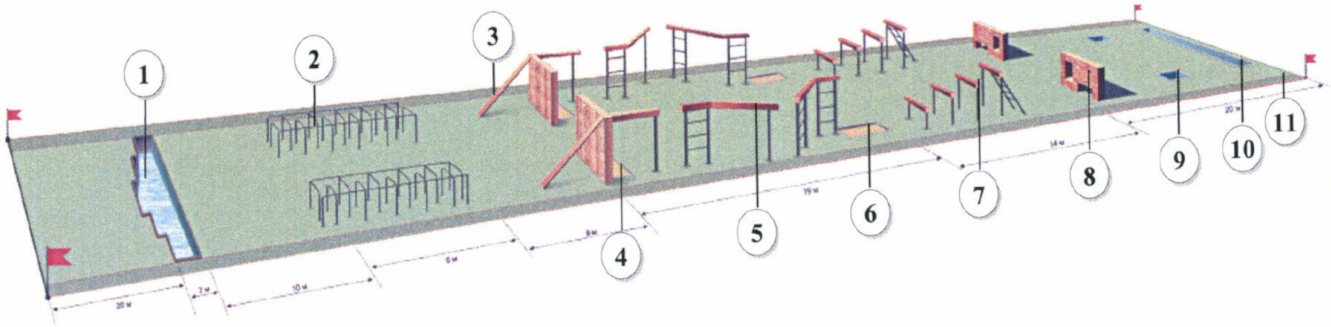
Рис. 43. Схема единой полосы препятствий
