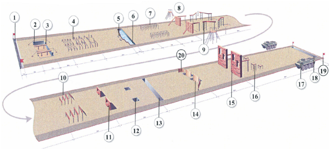
Рис. 44. Схема полосы препятствий Сухопутных войск и морской пехоты
