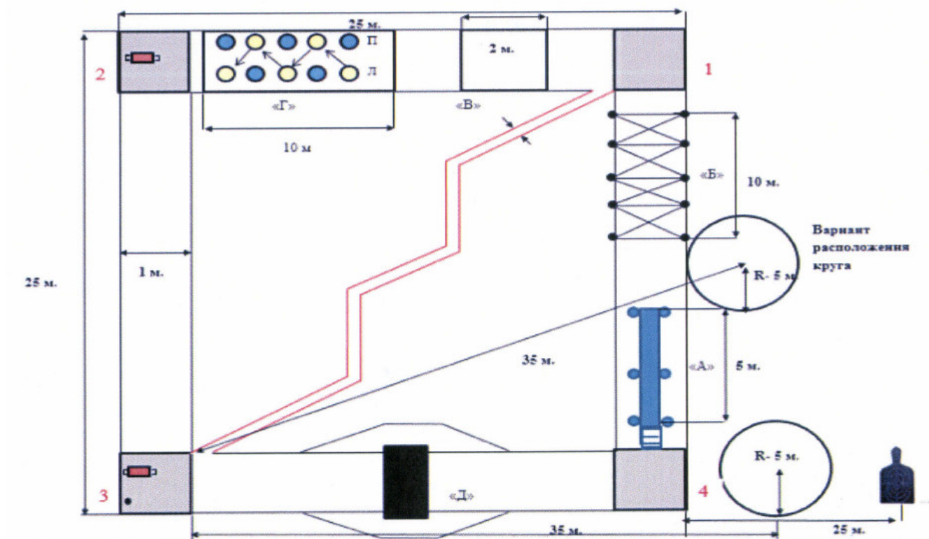
Рис. 91. Схема комплексного упражнения "Квадрат"
