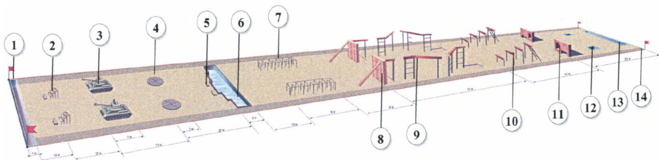
Рис. 45. Схема танковой полосы препятствий
