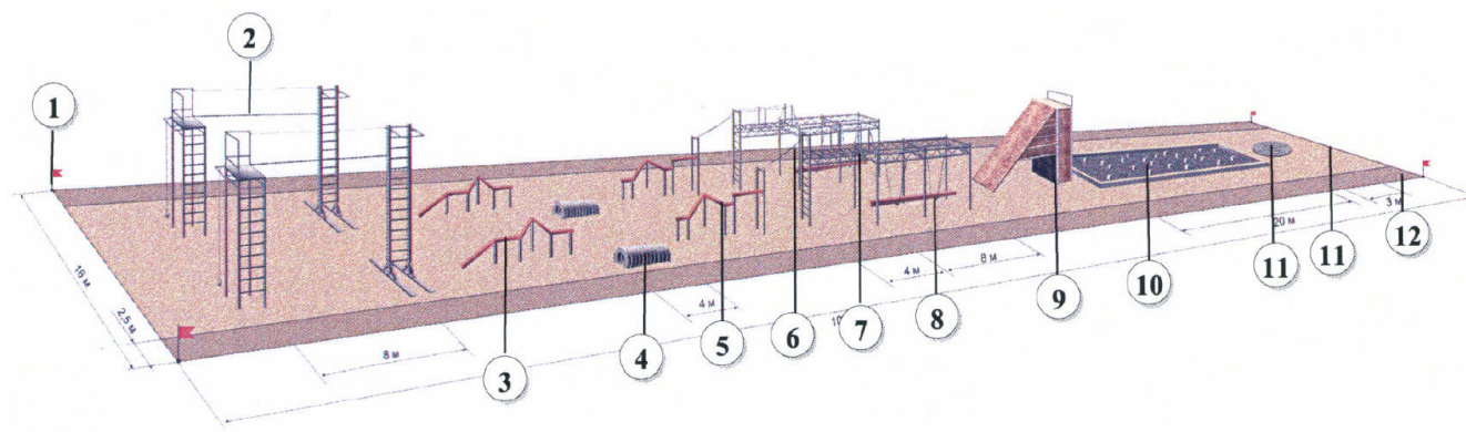
Рис. 48. Схема горной полосы препятствий
