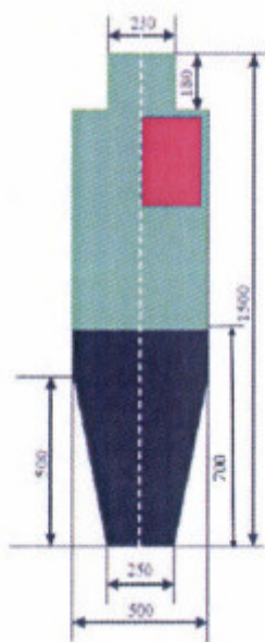
Рис. 86. Комбинированная мишень для выполнения метания ножа и малой пехотной лопаты на точность с места
