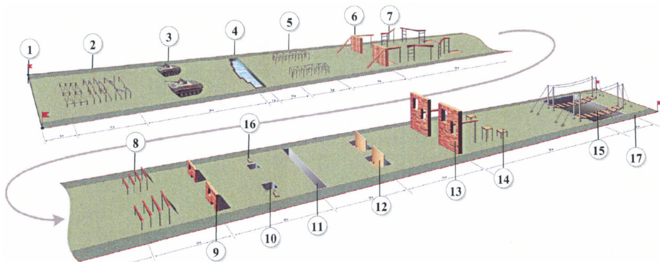
Рис. 46. Схема полосы препятствий Воздушно-десантных войск
